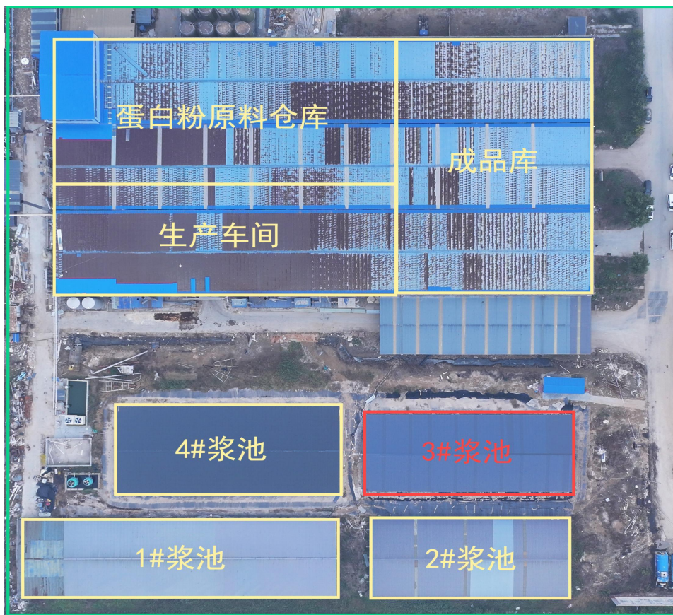
图1 厂区布局图
